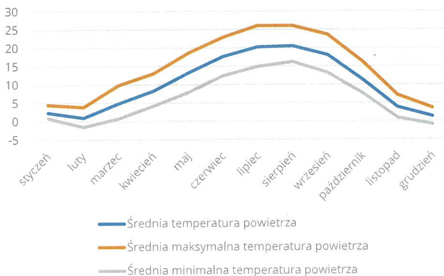
Wykres 2. Rozkład średniej miesięcznej temperatury powietrza w 2023 r. dla stacji synoptycznej IMGW Sandomierz (źródło: https://imgw.pl/ )
