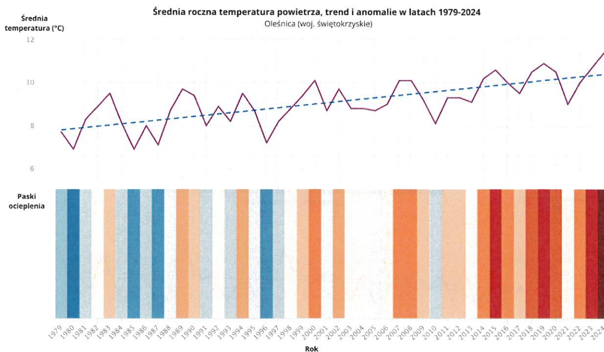
Wykres 3. Średnie roczne temperatury, trend oraz anomalie temperaturowe w latach 1979-2024 w Oleśnicy (Źródło: https://www.meteoblue.com/pl/pogoda/historyclimate/change/ole%c5% )
