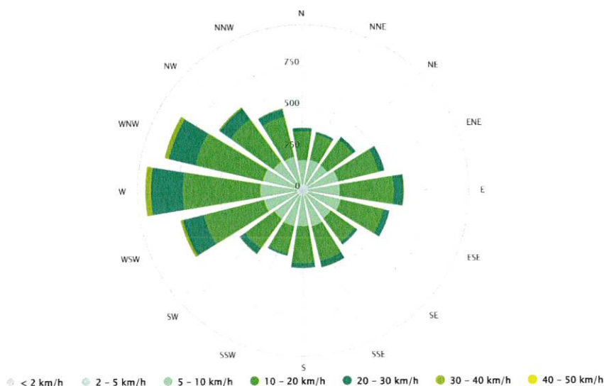
Rysunek 4. Róża wiatrów – Oleśnica (źródło:
